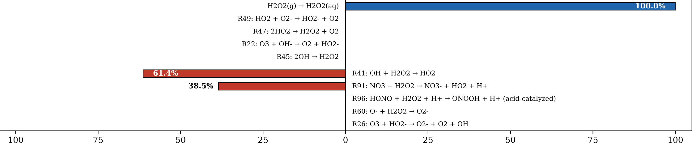
(d) \text{H}_2\text{O}_2 ( \Sigma\text{src} = 2.16\text{e-}08 \text{ M/s} )
